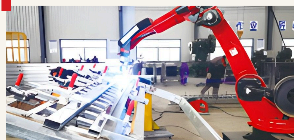
FOTOGRAFÍA · Planta en China · soldadura de marcos de acero
